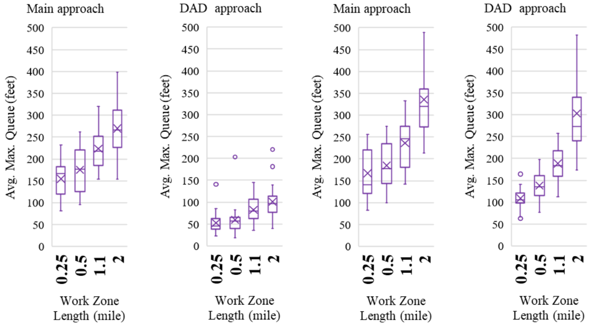
a. Queue for V_{Comb} of 50_25
