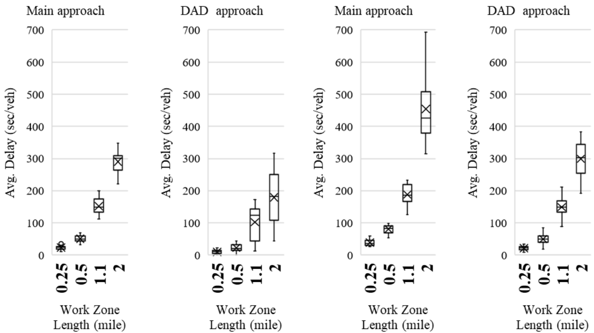
a. Delay for V_{Comb} of 50_25
