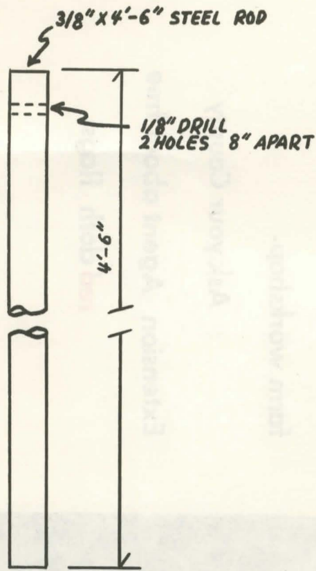
UPPER ROD
