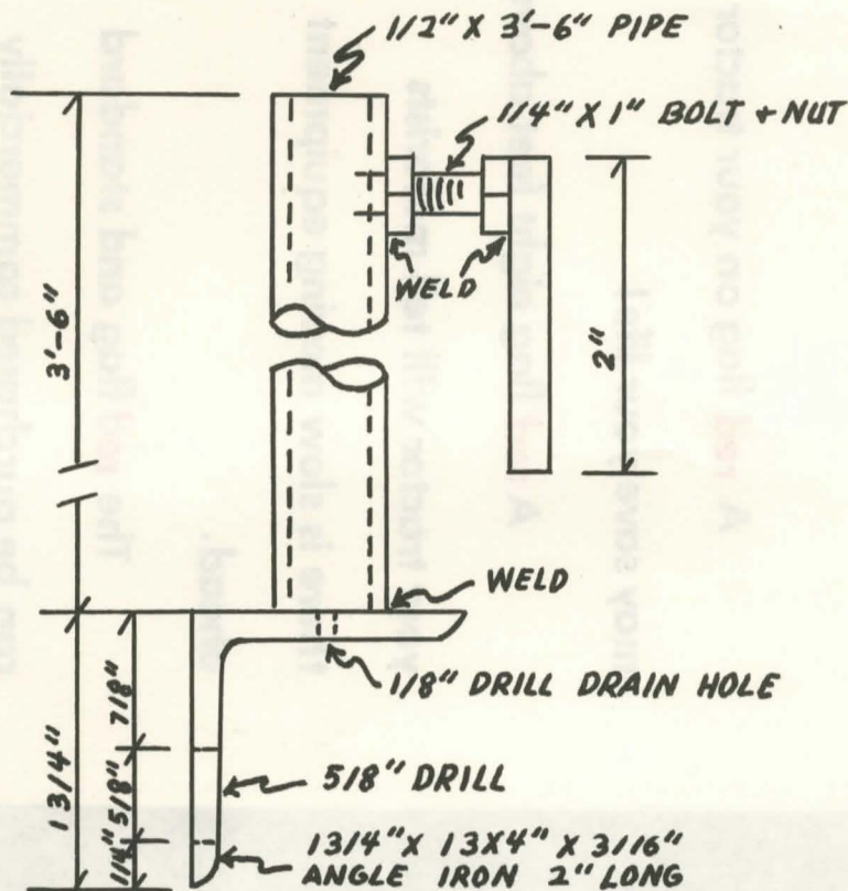
LOWER ROD
